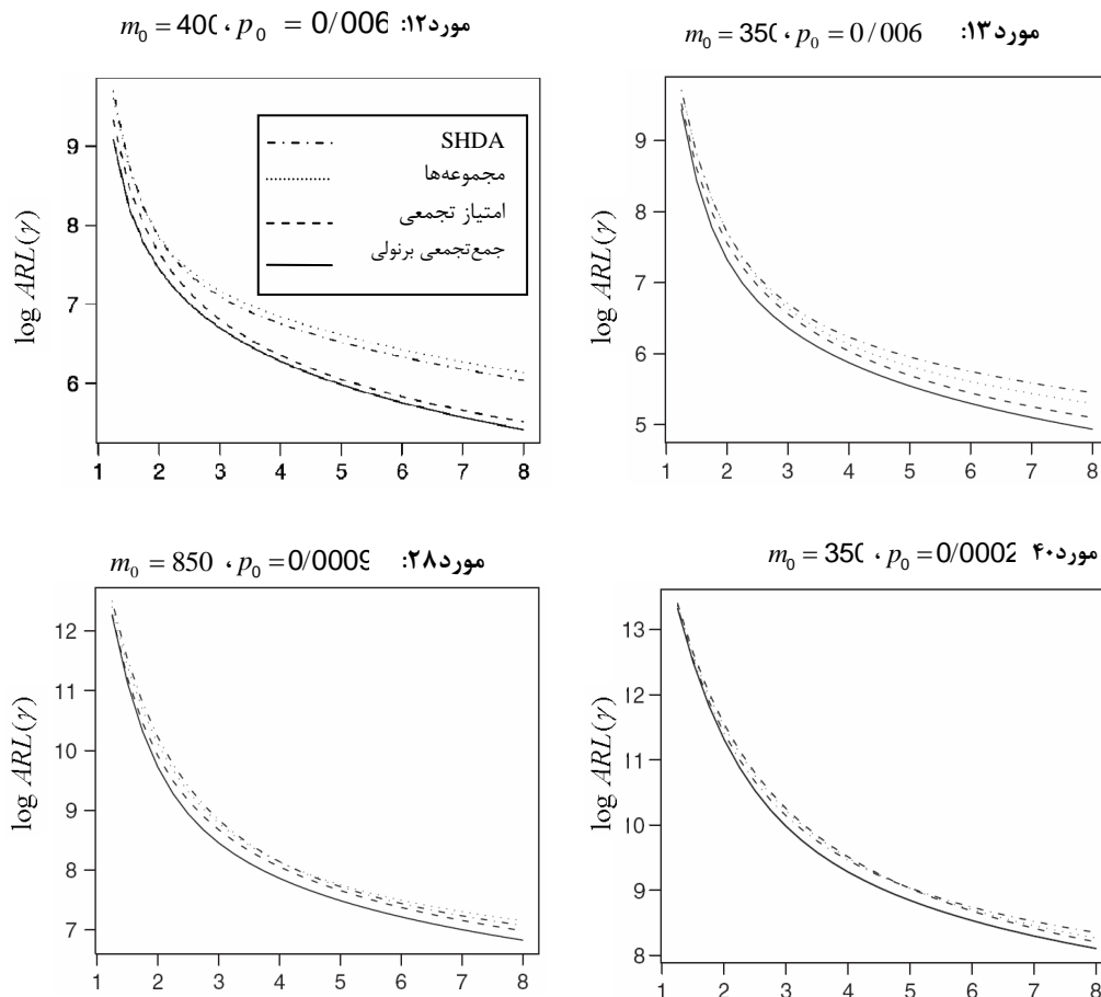
شکل ۱. مقایسه عملکرد چهار روش آماری به‌زای تغییرات مختلف (بر حسب \gamma ، ضریبی از p_0 ) برای موارد ۱۲، ۱۳، ۲۸ و ۴۰
