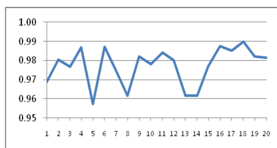
شکل ۴. نسبت مقدار شاخص SSE برای روش پیشنهادی به مقدار این شاخص برای روش k-prototypes بهبود یافته؛ مجموعه داده‌های ۲۰۰۰ تایی
