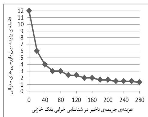
شکل ۵. فاصله‌ی بهینه بین بازرسی‌های متوالی بانک خازنی به ازاء مقادیر مختلف هزینه‌ی جریمه
