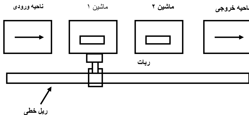
شکل ۱. طرح استقرار در سلول رباتیک دو ماشین
