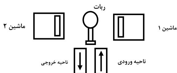
شکل ۲. سیکل پیشنهادی حرکات ربات در سلول دو ماشینیه
