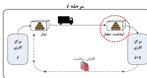
شکل ۳. جریان قطعات نیمه‌ساخته و کانبان برداشت در مرحله i
