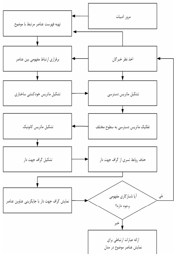
نمودار ۱. الگوریتم استخراج شبکه ارتباط عناصر طبق رویکرد ISM
