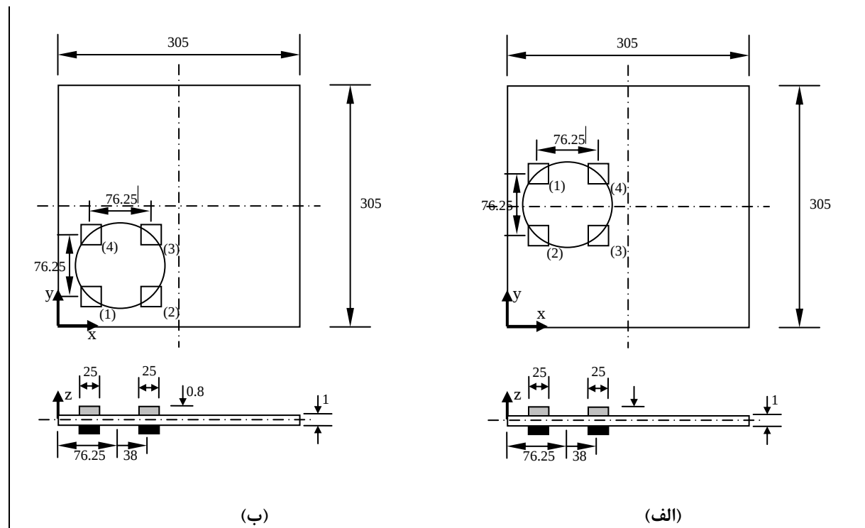
شکل ۳. آرایش ۴ تایی وصله‌ها در اطراف نقطه (الف) (l_x/4, l_y/2) (ب) (l_x/4, l_y/4)
