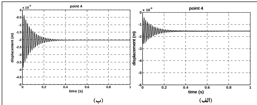
شکل ۴. جایابی عرضی نقطه (l_x/4, l_y/2) در مسئله اول
