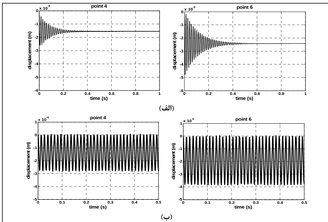
شکل ۵. جایابی عرضی نقطه (l_x/4, l_y/2) و (3l_x/4, l_y/2) در آرایش ۴ وصله تحت بارگذاری مسئله اول
