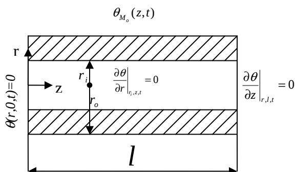
شکل ۱. استوانه توخالی همراه شرایط مرزی
