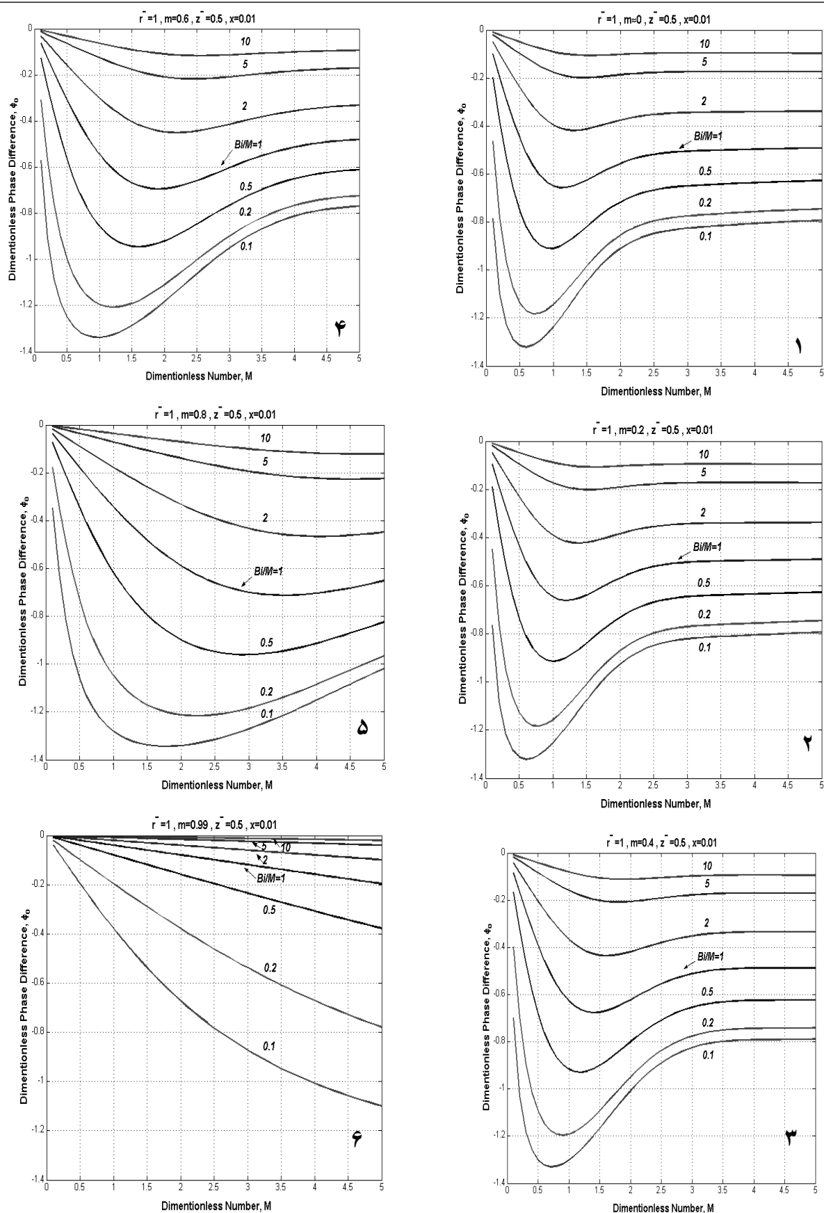
شکل ۶-۱ الی ۶-۶. نمودار تغییرات فاز بر حسب عدد بی بعد m
