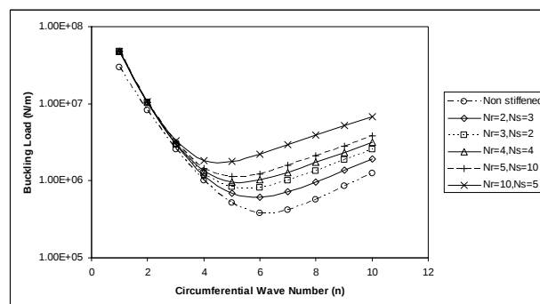
شکل ۳. اثر تعداد رینگها و استرینگرها بر بار کمانش پوسته دو سر ساده
