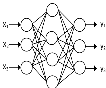
شکل ۲. شبکه عصبی سه لایه پیشخور
