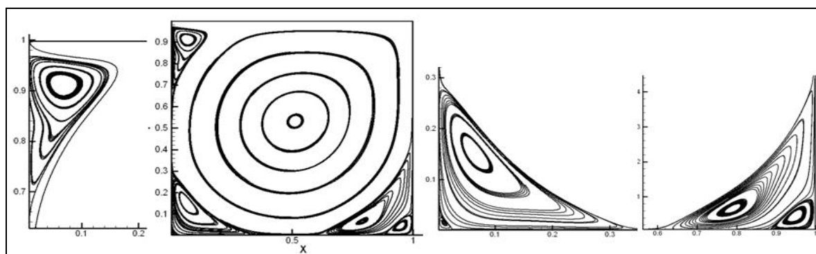
شکل ۱۴. خطوط جریان گردابه های اولیه و ثانویه و نمای بزرگ شده گردابه ها در Re=7500 .
