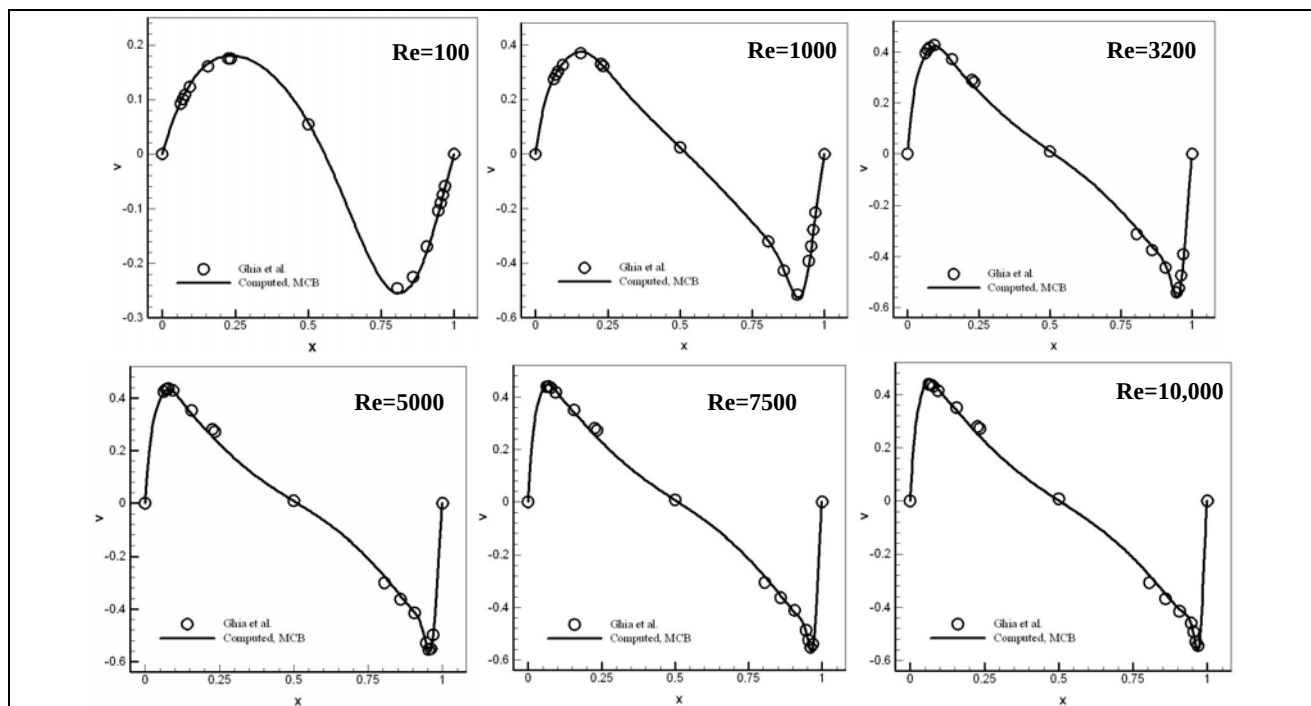
شکل ۱۹. مقایسه مقادیر محاسبه شده برای مولفه سرعت v در روی خط افقی گذرا از مرکز حفره با نتایج مرجع [27] Ghia et al. در اعداد رینولدز مختلف.
