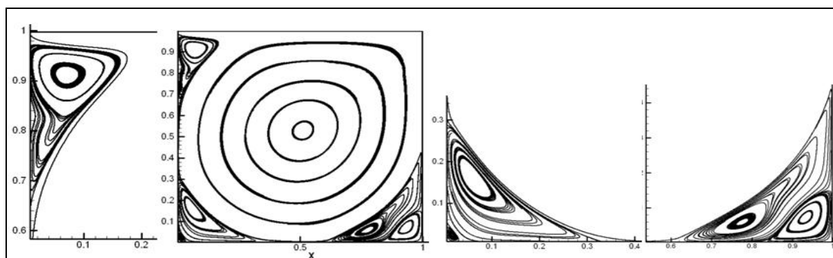
شکل ۱۵. خطوط جریان گردابه های اولیه و ثانویه و نمای بزرگ شده گردابه ها در Re=10,000 .
