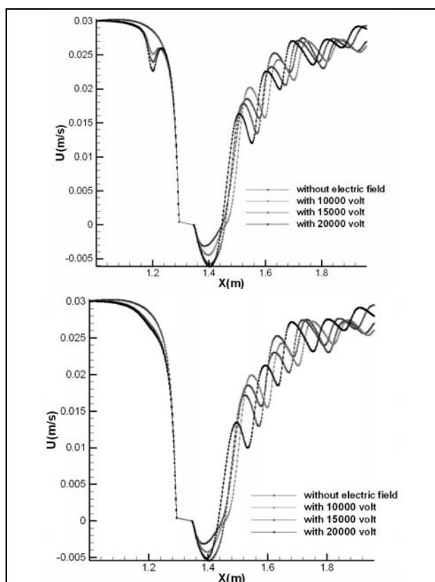
شکل ۱۲. پروفیل سرعت در امتداد خط مرکزی افقی کانال در
