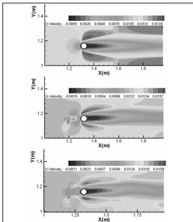
شکل ۶. کانتور سرعت در حالت‌های بدون ولتاژ (شکل اول)
