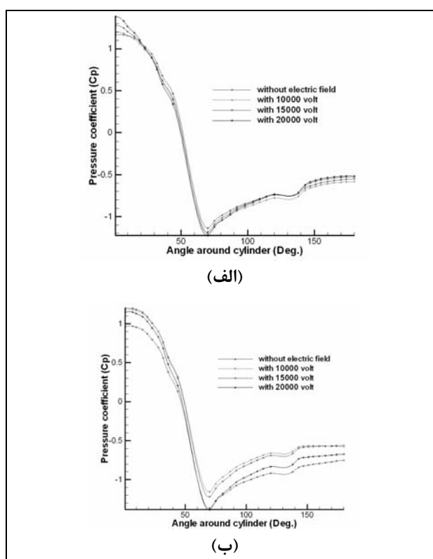
شکل ۱۰. نمودار مقایسه ضرایب فشار در نیمه بالایی استوانه
