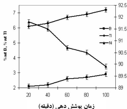
شکل ۴. تاثیر زمان پوشش دهی روی درصد وزنی نیکل، بُر و تالیوم در پوشش
