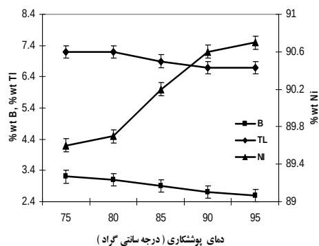
شکل ۷. تاثیر دمای پوشش دهی روی درصد وزنی نیکل، بر و تالیم پوشش در مدت زمان یکساعت.
