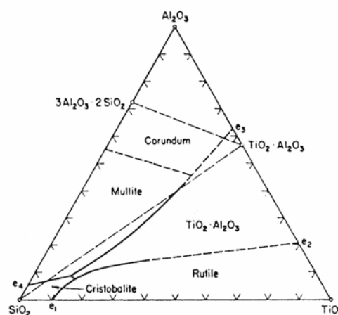
شکل ۱۴. دیگرام فازی تعادلی سه جزئی \text{TiO}_2 - \text{SiO}_2 - \text{Al}_2\text{O}_3 [۱۳]
