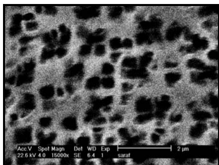
شکل ۹. عملیات محلول سازی (۱۱۰۰°C / ۴۰ MPa/۹h/AC)
