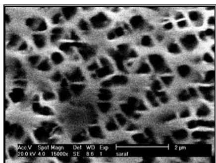
شکل ۱۱. عملیات محلول سازی (۱۱۰۰°C / ۸۰ MPa/۱۱h/AC)
