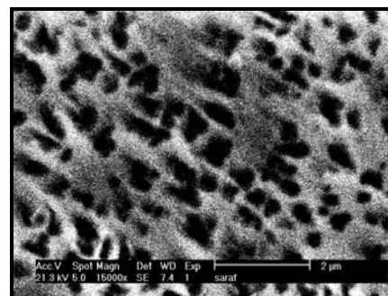
شکل ۸. عملیات محلول سازی (۱۱۰۰°C / ۲۰ MPa/۸h/AC)
