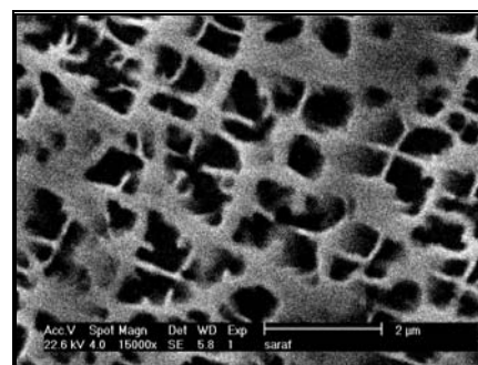
شکل ۱۰. عملیات محلول سازی (۱۱۰۰°C / ۶۰ MPa/۱۰h/AC)
