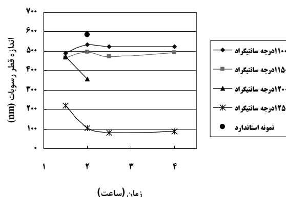
شکل ۶. نمودار میانگین اندازه قطر رسوبات درون دانه ای بر حسب زمان در دمای ثابت
