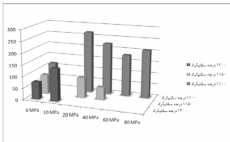
شکل ۱۲. نمودار مقایسه ای تعداد رسوب در 100\mu m^2 بر حسب دما و میزان تنش اعمالی
