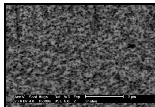
شکل ۳. عملیات محلول سازی (۱۱۲۵°C/۲.۵h/AC) های ثانویه
