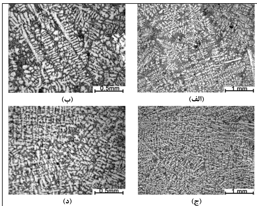
شکل ۷. ساختار میکروسکوپی نمونه‌های (الف) و (ب) A، (ج) و (د) G. مشاهده می‌شود که با افزایش فرکانس و نزدیک شدن به حد تثویک بحرانی در نقشه فرکانس-دامنه، رشد و ساختار دندریتی از بین رفته و علاوه بر آن، فاز یوتکتیک Al-Si بصورت همگن در فضای بین دندریتی جای گرفته است.
