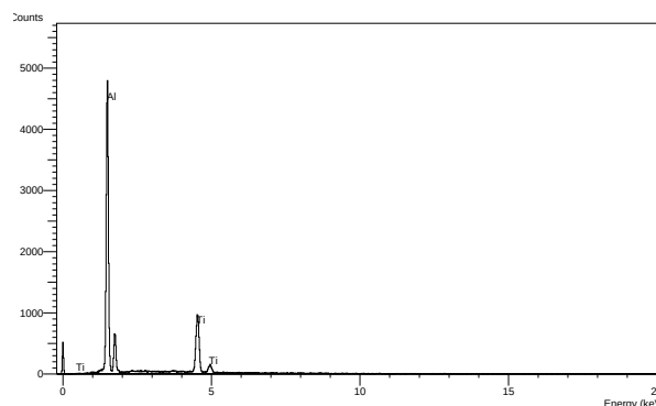
شکل ۳. آنالیز EDS زمینه آلومینیومی مجاور به ذرات پودر
