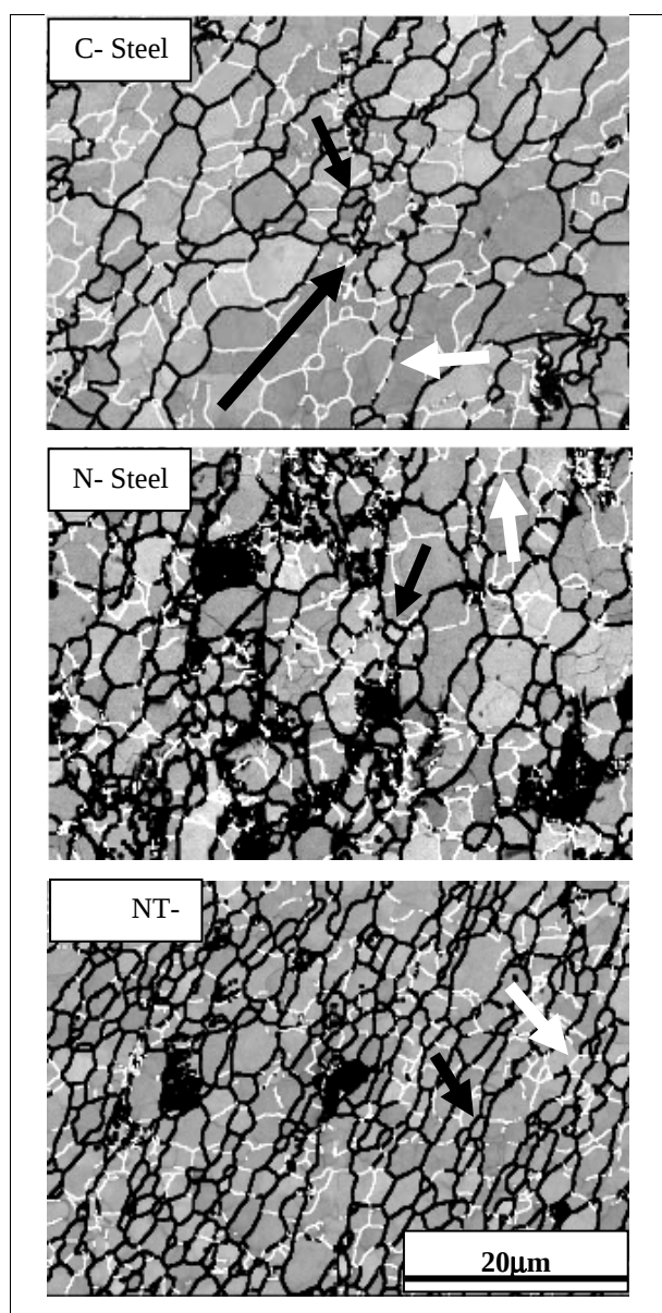
شکل ۵. نتایج EBSD فولادهای C، N و NT در شرایط تغییر شکل داده شده تا کرنش ۲ و با نرخ کرنش 1 \times 10^{-1} \text{ s}^{-1} در منطقه دو فاز.
