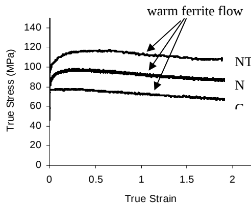
شکل ۲. منحنی های تنش-کرنش در تغییر شکل فریت در فولادهای C، N و NT تا کرنش ۲ و با نرخ کرنش 0.01 \text{ s}^{-1} .
