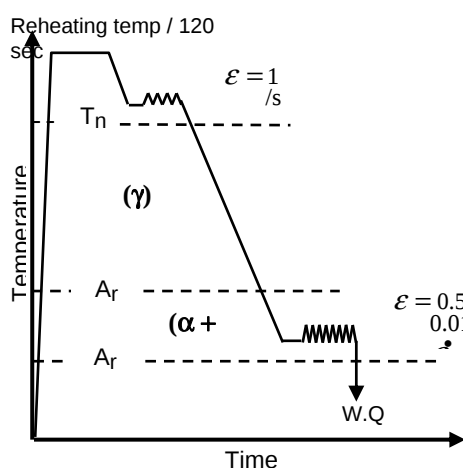
شکل ۱. برنامه عملیات ترمومکانیکی آزمایش پیچش گرم اجرا شده بر روی فولادهای مورد تحقیق.
