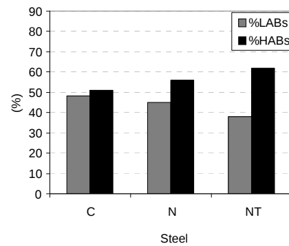
شکل ۶. درصد LABs و HABs در فولادهای C، N و NT در شرایط تغییر شکل تا کرنش ۲ و با نرخ کرنش 1 \times 10^{-1} s^{-1} در منطقه دو فازی.
