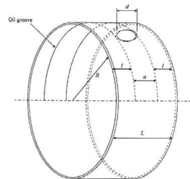
شکل ۱. یاتاقان با شیار محیطی [۷]
