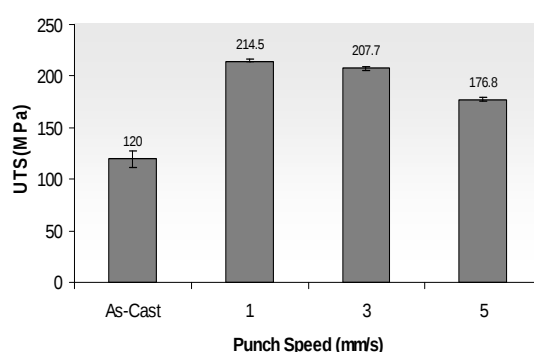
شکل ۱۰. تغییرات استحکام کششی بر حسب سرعت پانچ
