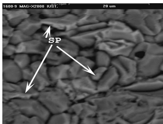
شکل ۷. تصویر ریزساختاری نمونه حاوی ۹ درصد \text{TiO}_2 پخته شده در دمای (1600^\circ\text{C}/2\text{h}) در بزرگنمایی (\times 2000)
