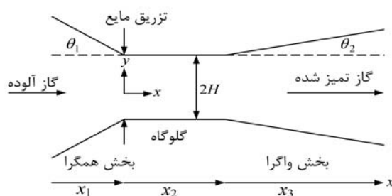
شکل ۱. شماتیک یک شوینده و نتوری
