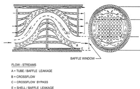
شکل ۳. جریان‌های مؤثر سمت پوسته طبق مدل تینکر [۴]
