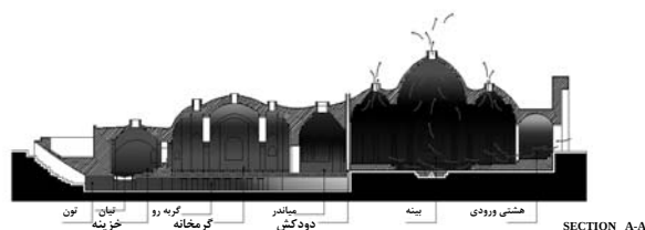
شکل ۴. نحوه تجمع حرارت در گرمابه کردشت [۶]
