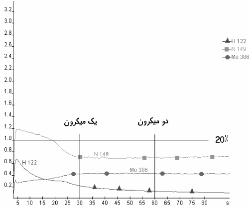
نمودار ۷-۳. فولاد ۳۱۶ پس از ۵ ساعت پرتو دهی
