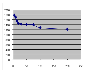
نمودار ۱-۳. افزایش طول رنجیره مارکوف و بررسی تاثیر آن بر متوسط فاصله از جواب‌های موثر
