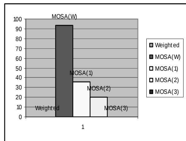
نمودار ۳-۷. مقایسه متوسط فاصله از جواب های موثر برای مساله 10 \times 10 با روش دقیق و شبیه سازی تبرید
