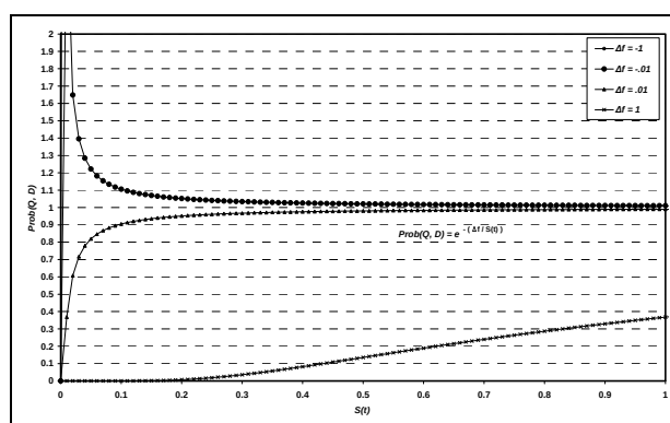
شکل ۱. نحوه تغییرات احتمال انتخاب زنبورهای نر بر حسب تغییرات سرعت
