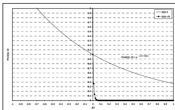
شکل ۲. نحوه تغییرات احتمال انتخاب زنبورهای نر بر حسب تغییرات اختلاف مقدار تابع هدف
