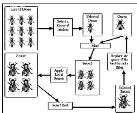
شکل ۳. الگوریتم HBMO [۲]
