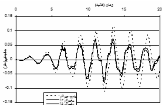
شکل ۱۸. جابجایی نقطه ای از بام در سازه میرا (ξs = ۵٪)
