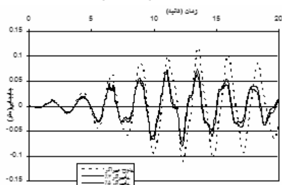
شکل ۱۸. جابجایی نقطه ای از بام با در سازه میرا ( \xi_s = 0.5\% ) تحت زلزله منجیل (آب بر)
