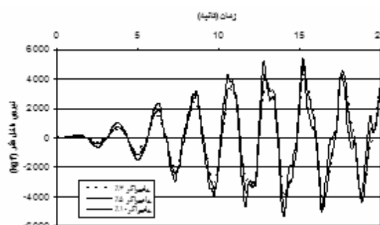
شکل ۱۶. مقدار نیروی فتر در سازه نامیرا تحت زلزله منجیل
