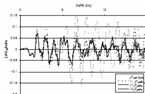
شکل ۲۵. جابجایی نقطه‌ای از بام تحت زلزله السنتر
