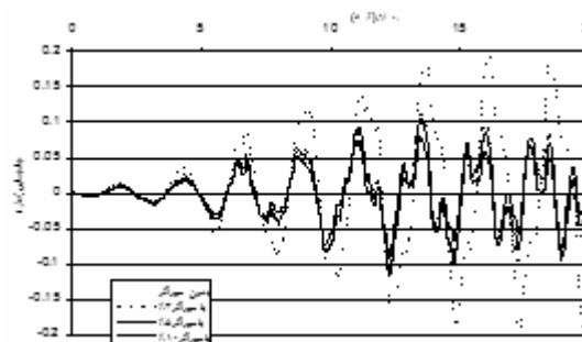
شکل ۲۹. جابجایی نقطه‌ای از دیافراگم بام هنگامیکه میراگر در طبقه ۶ قرار داشته باشد (تحت زلزله منجیل)
