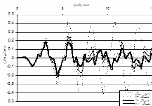
شکل ۲۸. جابجایی نقطه‌ای از دیافراگم بام هنگامیکه میراگر در طبقه ۶ قرار داشته باشد (تحت زلزله السنترو)
