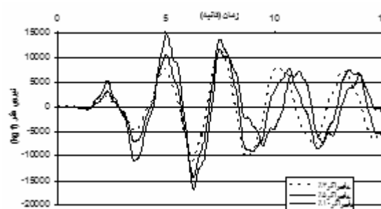
شکل ۱۵. مقدار نیروی فتر در سازه نامیرا تحت زلزله السنترو
