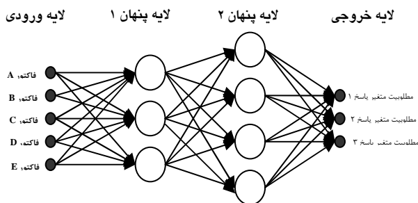
شکل ۵. شبکه عصبی استفاده شده با تعداد نرونهاي ۳ و ۴ در لایه های پنهان اول و دوم
