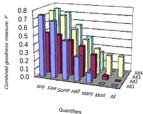
شکل ۲. امتیاز نهایی هر گزینه با کمک روش Borda-OWA
