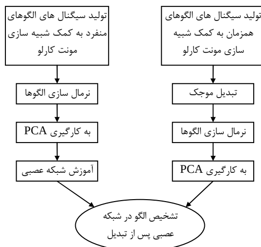
شکل ۲. ساختار کلی روش پیشنهادی
