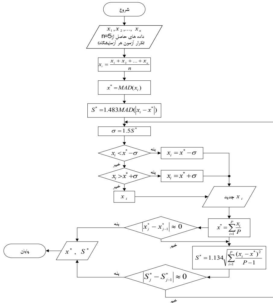
شکل ۲. فلوچارت روش آماری استوار در آزمون مهارت سیم و کابل
