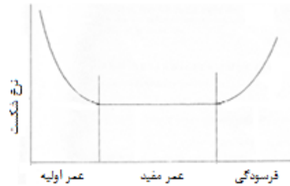
شکل ۱. منحنی میرایی
