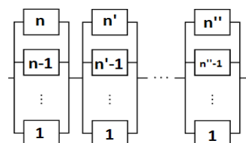
شکل ۲. شمای کلی یک سیستم سری-موازی
