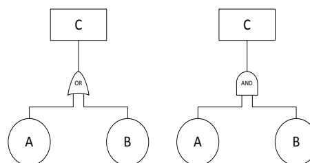
شکل ۵. درخت خرابی مربوط به گره های A, B, C با دریاچه های And و OR
