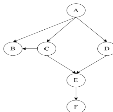
شکل ۴. شبکه بیزین فرضی
