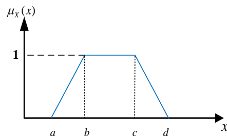
شکل ۳. تابع عضویت یک عدد فازی ذوزنقه ایی
