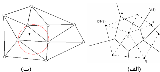
شکل ۷. (الف) مثلث بندی دلونی (خط چین) به همراه دوگان وُرونویی آن؛ (ب) نمایش خاصیت سوم مثلث بندی دلونی
