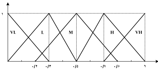
شکل ۲. توابع عضویت متغیرهای کلامی مجموعه W
