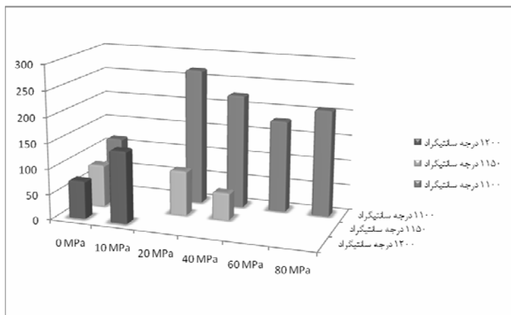
شکل ۱۲. نمودار مقایسه ای تعداد رسوب در ۱۰۰ μm ۲ بر حسب دما و میزان تنش اعمالی
