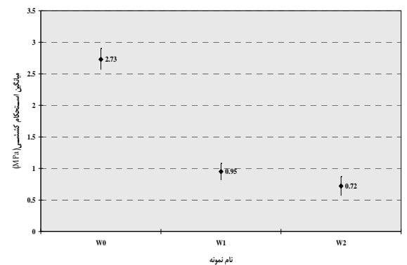
شکل ۱۰. تأثیر عملیات تصفیه بر اندیس چگالی نمونه‌های آلیاژ ۶۰۶۳
