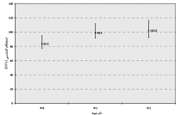
شکل ۸. نمودار استحکام کششی نمونه‌های مختلف آلیاژ ۶۰۶۳
