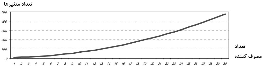
شکل ۶. نمودار افزایش تعداد متغیرها به ازای افزایش تعداد مصرف کننده‌ها در مدل (۶) تا (۱۲)
