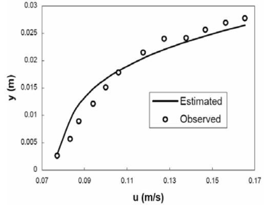
شکل ۳. مقایسه نتایج اندازه‌گیری شده و نتایج مدل برای یک نمونه آزمایش با مشخصات = ارتفاع نی، ۱۰ cm = عمق آب، ۶۷ mm = lit/s، دبی، ۴/۹۶۳ = شیب کف فلوم
