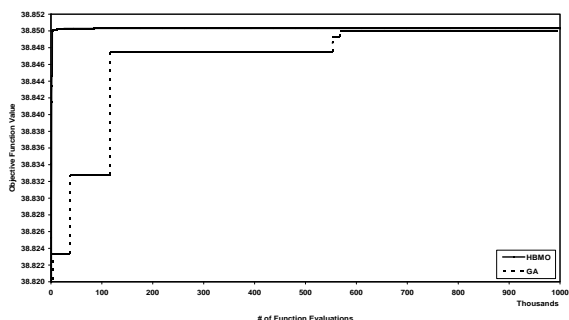
شکل ۷. تغییرات حداکثر مقدار تابع هدف در ۱۰ بار اجرا و در طول تعداد دفعات ارزیابی تابع
