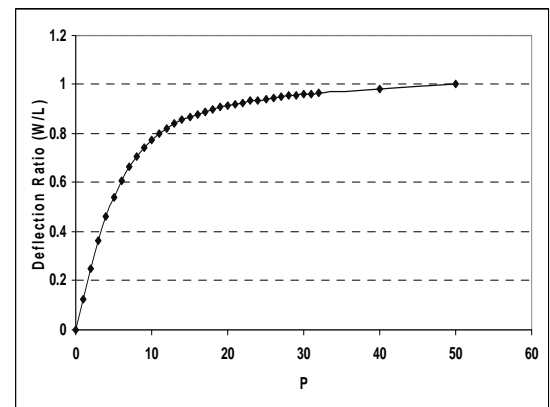
شکل ۳. رفتار کامل بار - خیز تیر
