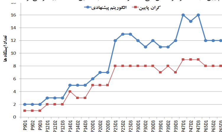
شکل ۳. تعداد ایستگاه‌های حاصل از الگوریتم و کران پایین ۳
