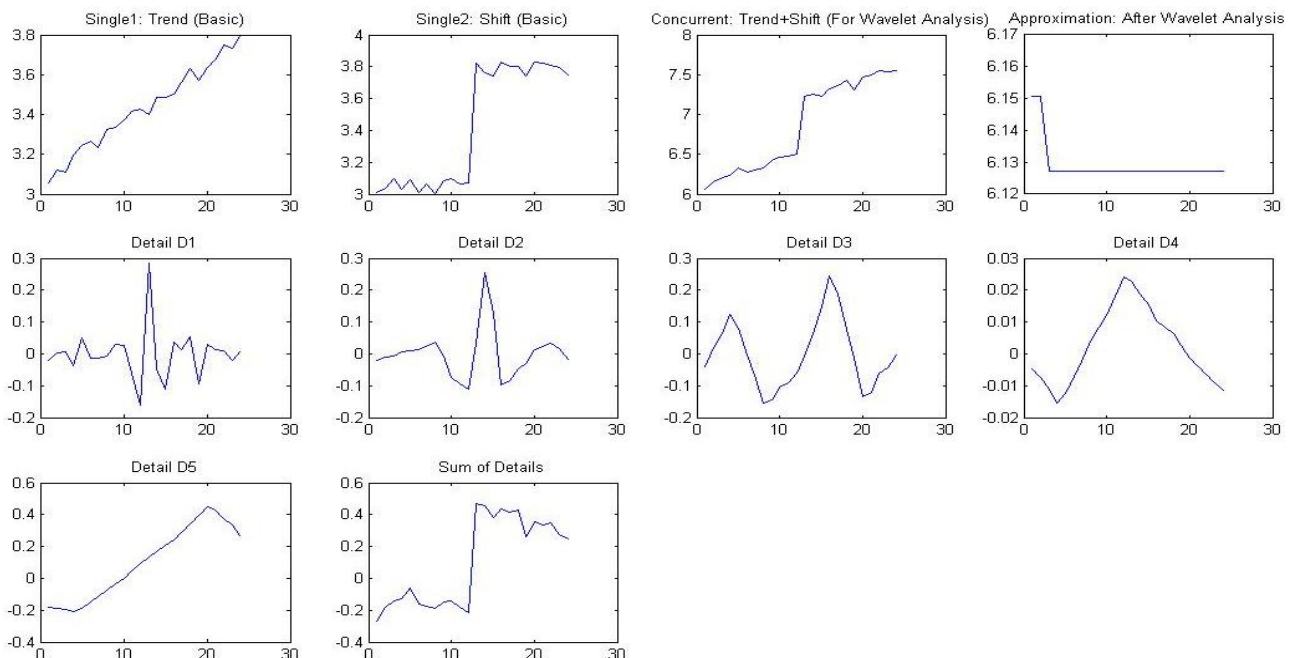
شکل ۴. مرحله اول تبدیل موجک (استخراج شیفت)
