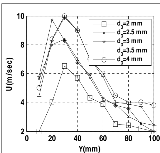
۱b. سرعت محوری قطرات با قطر خروجی نازل
