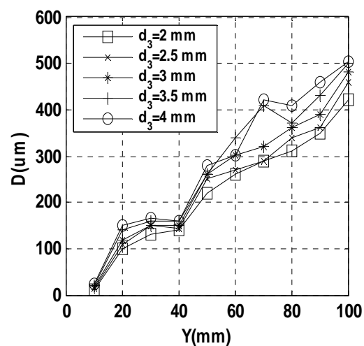
۱a. تغییرات اندازه قطرات با قطر خروجی نازل
