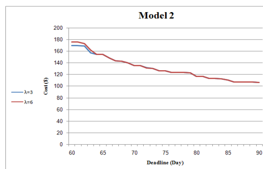
شکل ۳. نمودار زمان اتمام- هزینه در مدل ۲
