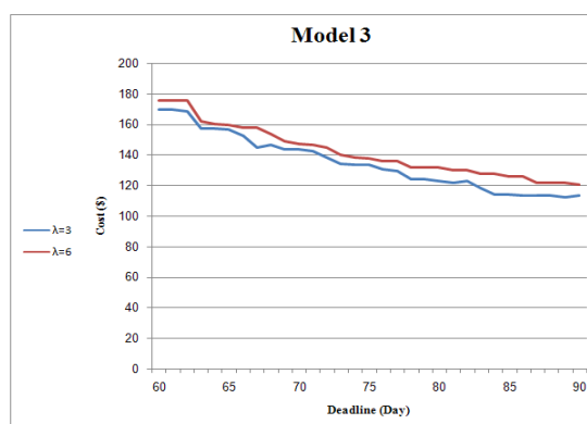
شکل ۴. نمودار زمان اتمام- هزینه در مدل ۳
