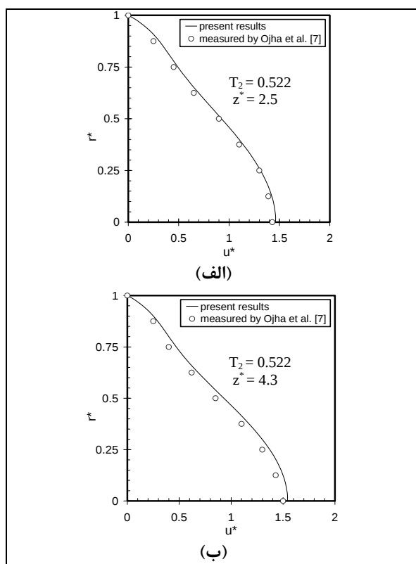
شکل ۷. پروفیل‌های سرعت محوری برای دو نقطه در طول لوله،
