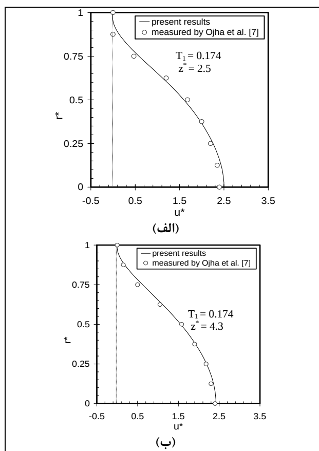
شکل ۶. پروفیل‌های سرعت محوری برای دو نقطه در طول لوله،
